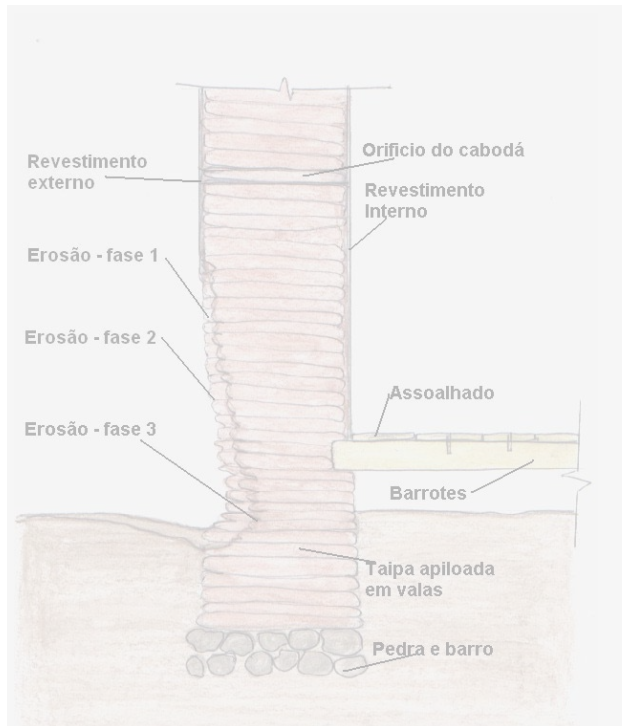
Figura 1 – Fases típicas de erosão das paredes de taipa
